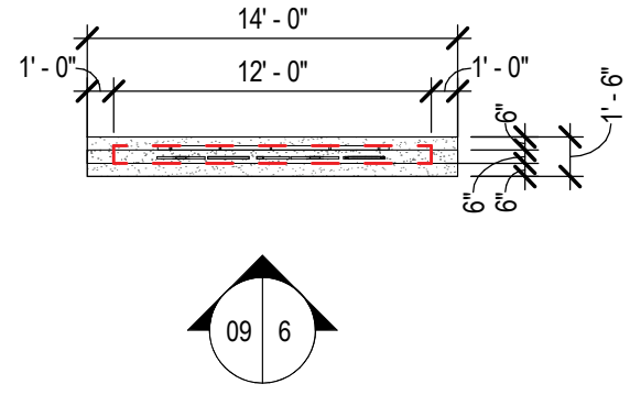
5 MONUMENT SIGN PLAN SCALE: 1/8" = 1'-0"
