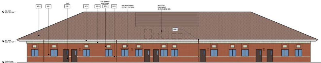
4 NORTH ELEVATION SCALE: 1/8" = 1'-0"
