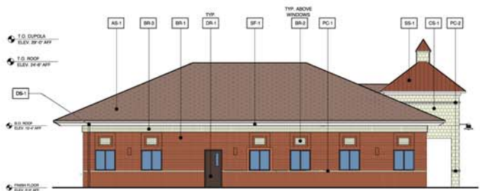
2 WEST ELEVATION SCALE: 1/8" = 1'-0"
