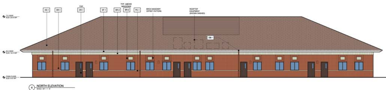
4 NORTH ELEVATION SCALE: 1/8" = 1'-0"
