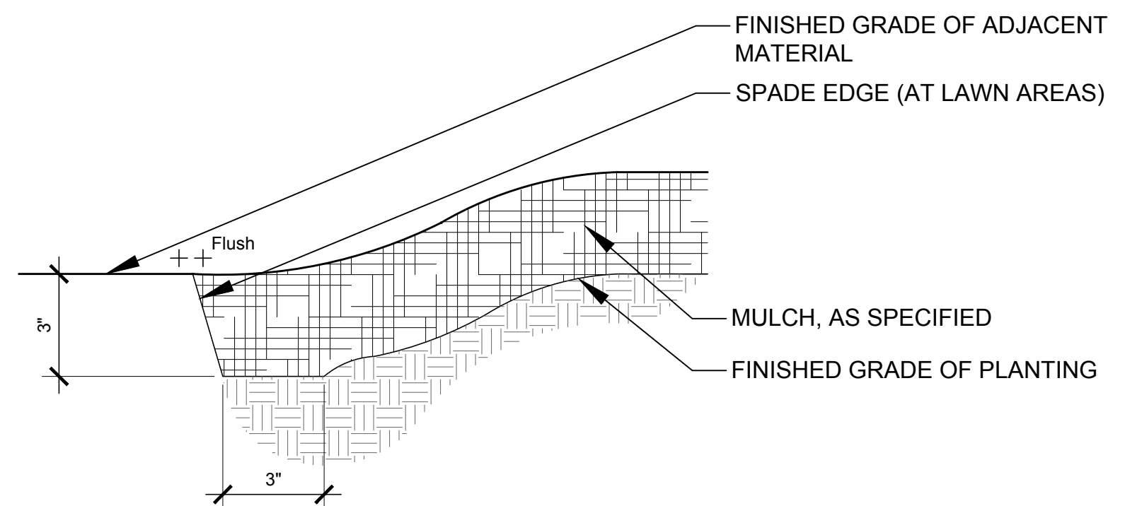
5 PLANTING BED EDGE Scale: 3" = 1'-0"
